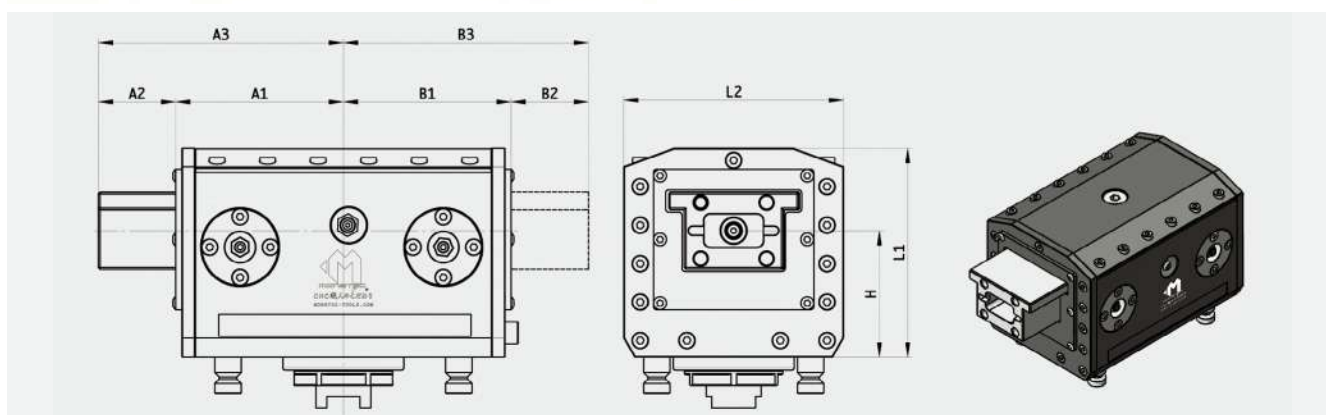
ブローチングユニット 寸法一覧（単位：mm）
